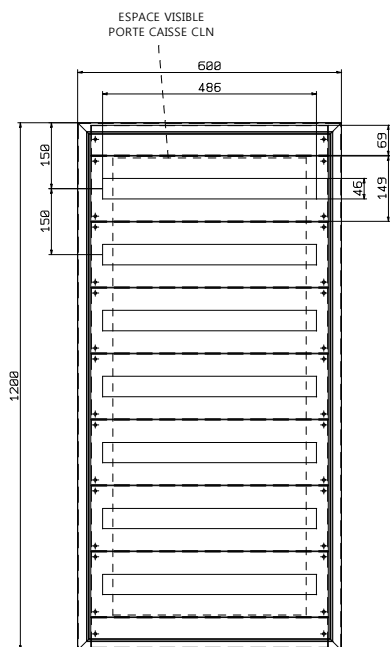
CLNMOD60120 LARGEUR DE MODULE=18mm TOTAL MODULES=7x27
