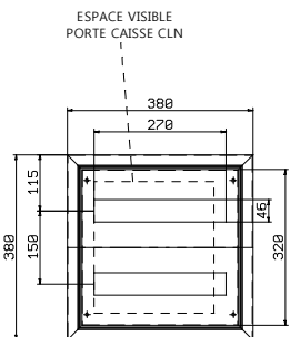
CLNMOD3838 LARGEUR DE MODULE=18mm TOTAL MODULES=2x15
