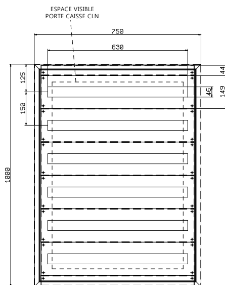
CLNMOD75100 LARGEUR DE MODULE=18mm TOTAL MODULES=6x35
