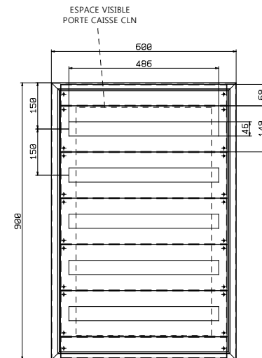
CLNMOD6090 LARGEUR DE MODULE=18mm TOTAL MODULES=5x27
