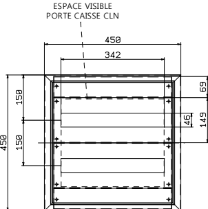
CLNMOD4545 LARGEUR DE MODULE=18mm TOTAL MODULES=2x19
