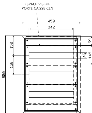
CLNMOD4560 LARGEUR DE MODULE=18mm TOTAL MODULES=3x19
