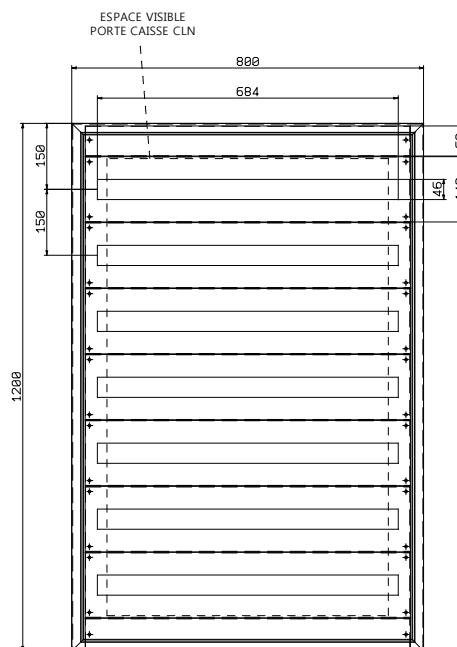
CLNMOD80120 LARGEUR DE MODULE=18mm TOTAL MODULES=7x38
