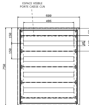
CLNMOD6075 LARGEUR DE MODULE=18mm TOTAL MODULES=4x27
