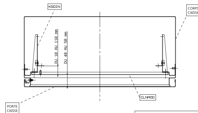
VUE DE SECTION CAISSE AVEC ACCESSOIRES
