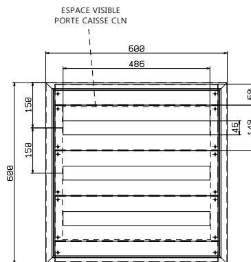
CLNMOD6060 LARGEUR DE MODULE=18mm TOTAL MODULES=3x27
