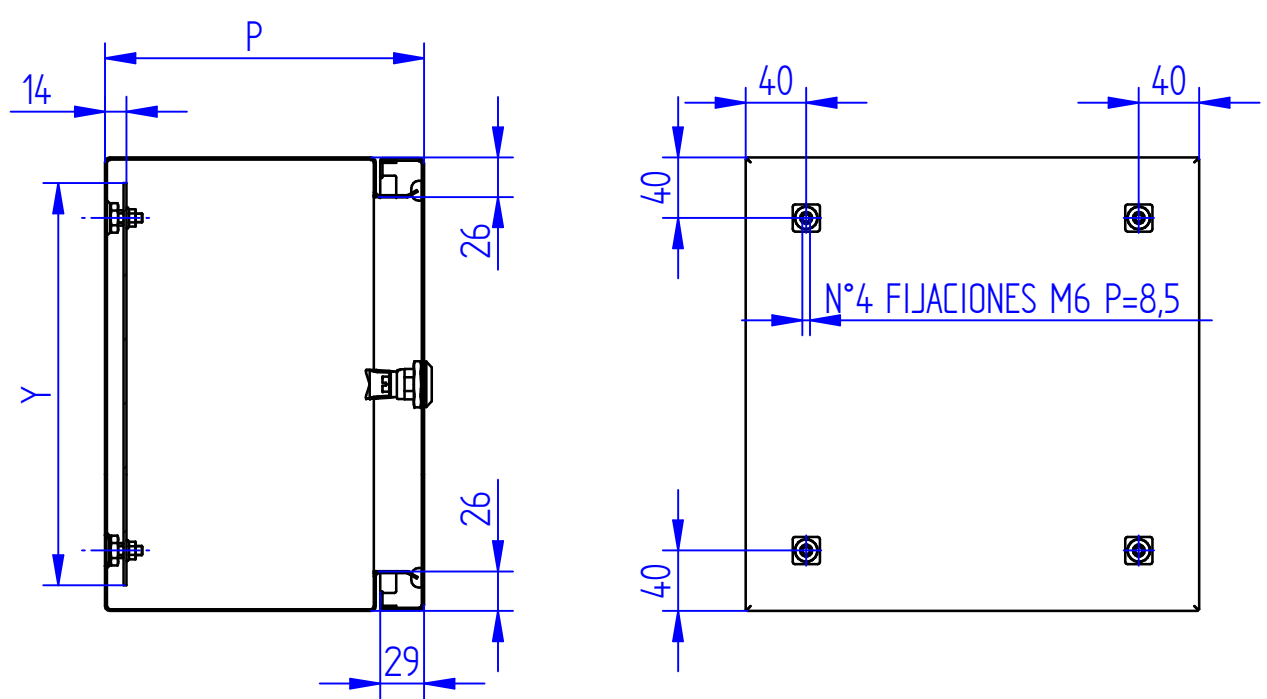
SECCIÓN D-D
