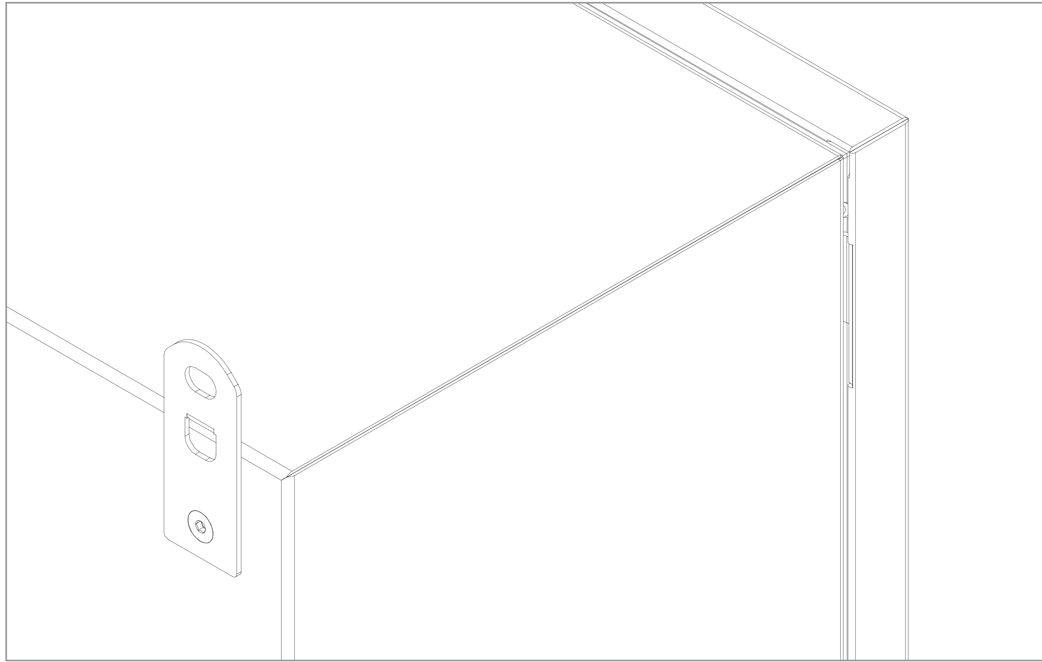
DETALLE POSTERIOR CAJAS CON ESTRIBO VERTICAL
