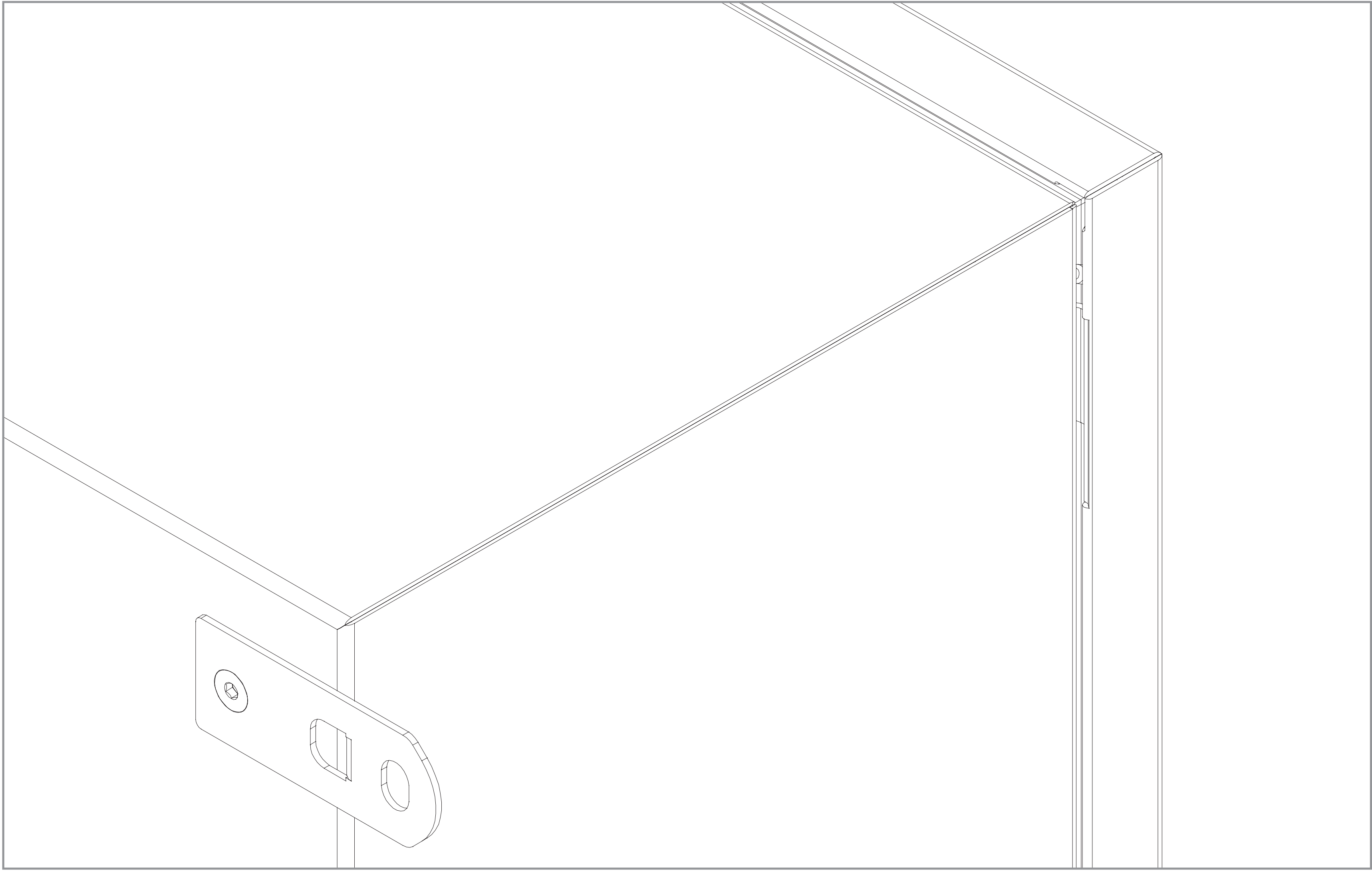
DETALLE POSTERIOR CAJAS CON ESTRIBO HORIZONTAL
