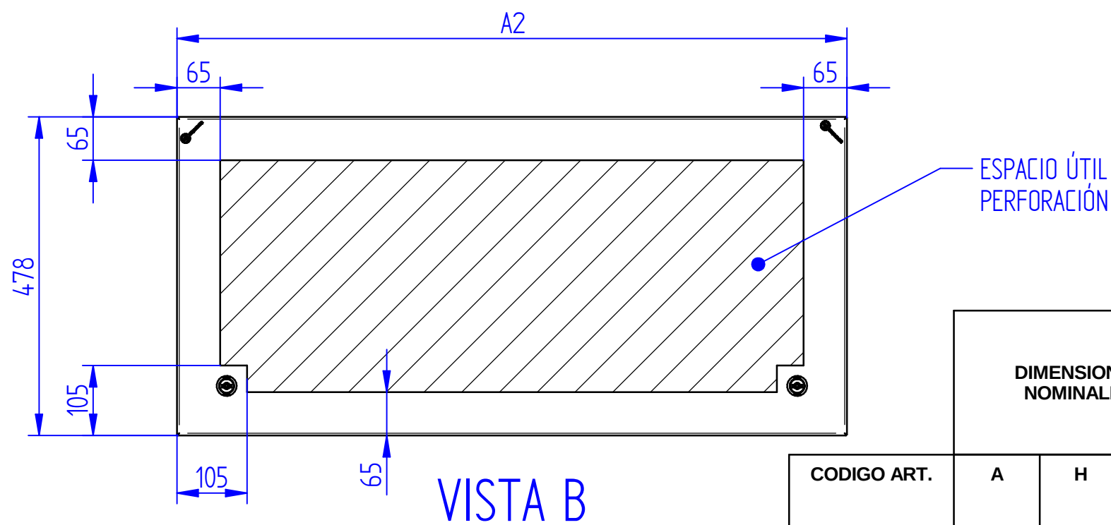
SECCIÓN A-A
