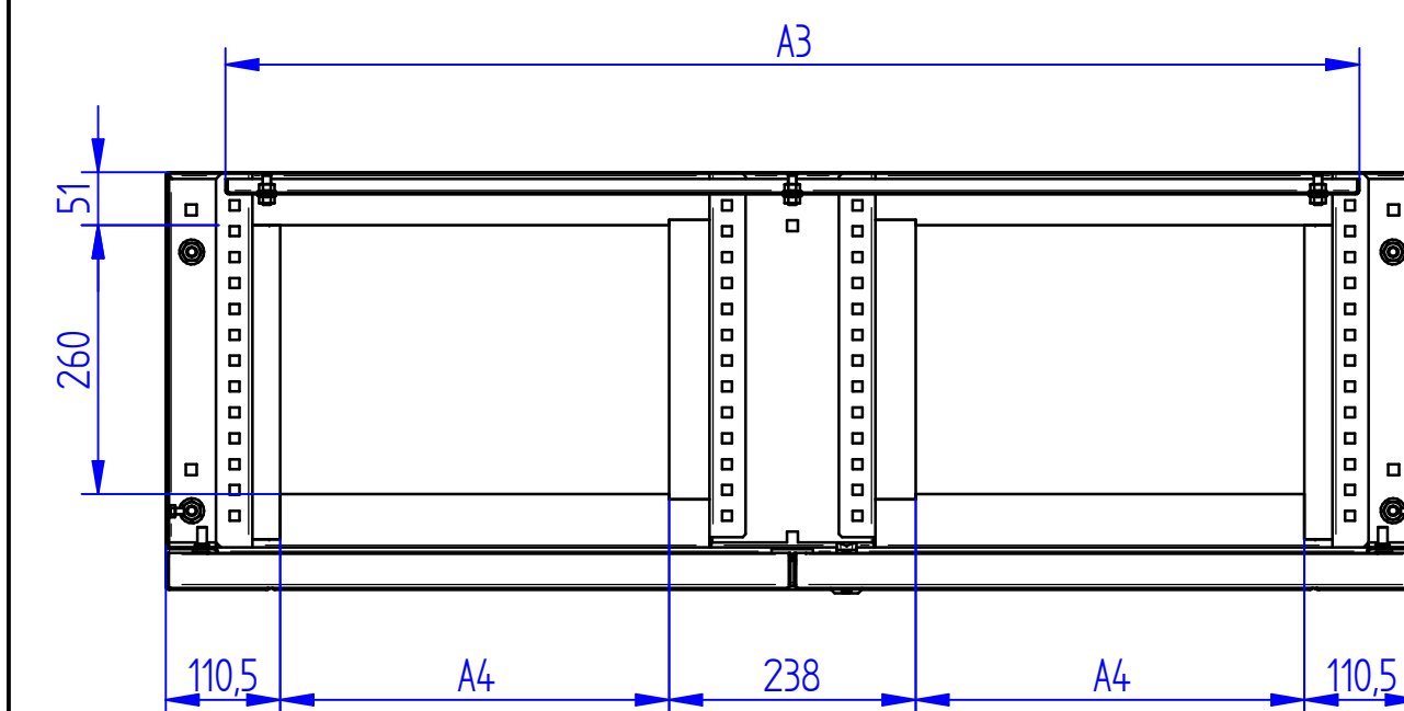
SECCIÓN C-C
