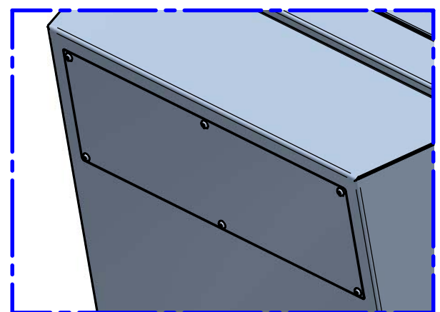
DETAIL MIT HINTEREN STANDARD-FLANSCHES
