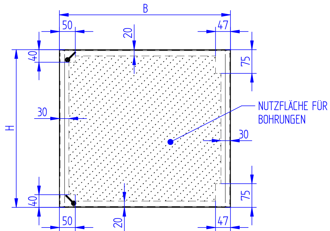
DETAIL DES HINTEREN STANDARD-FLANSCHES
