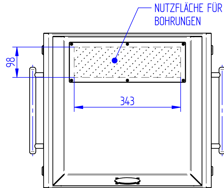
DETAIL DES HINTEREN STANDARD-FLANSCHES
