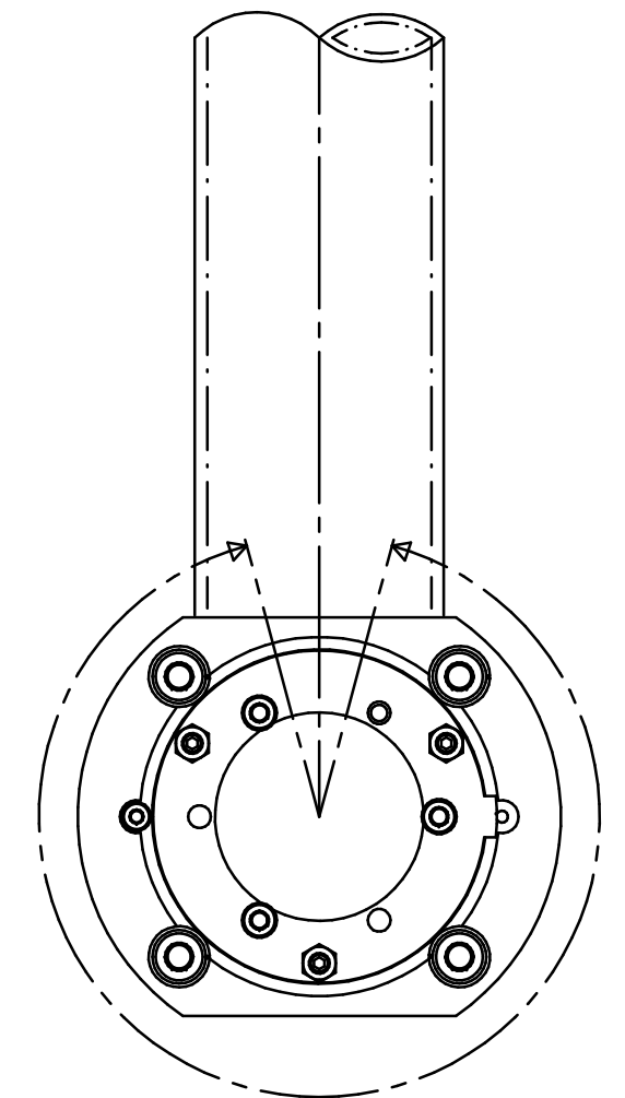
330° STEUERGEHÄUSE SEITE
