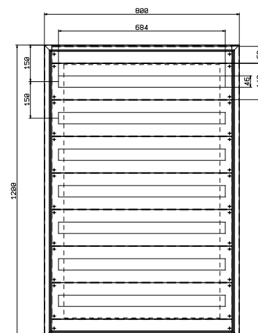
CLNMOD80120 266 MODULES
