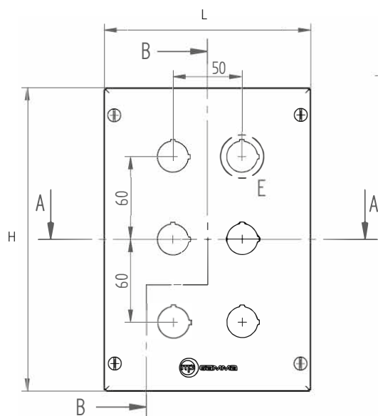
VUE FRONTAL
