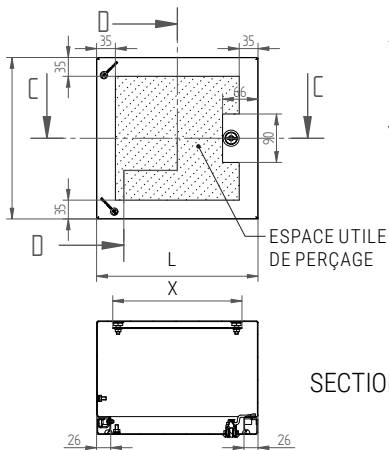
VUE FRONTAL
