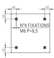
VUE ARRIÈR
