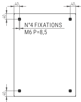
VUE ARRIÈR
