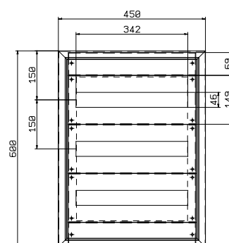
CLNMOD4560 57 MODULES
