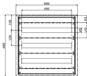
CLNMOD6060 81 MODULES
