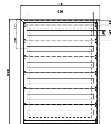
CLNMOD75100 210 MODULES
