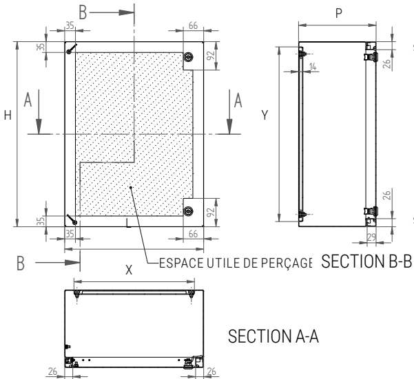
VUE FRONTAL
