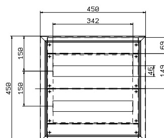
CLNMOD4545 38 MODULES
