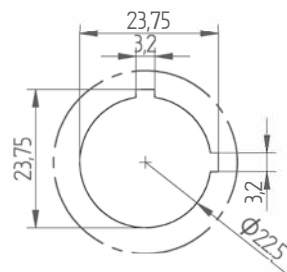
DÉTAIL E
