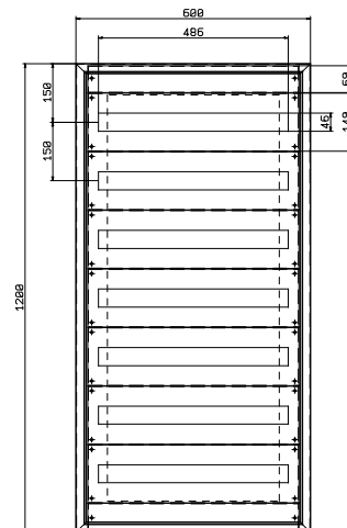
CLNMOD60120 189 MODULES
