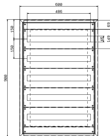
CLNMOD6090 135 MODULES
