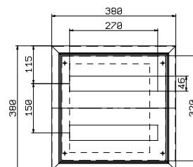
CLNMOD3838 30 MODULES
